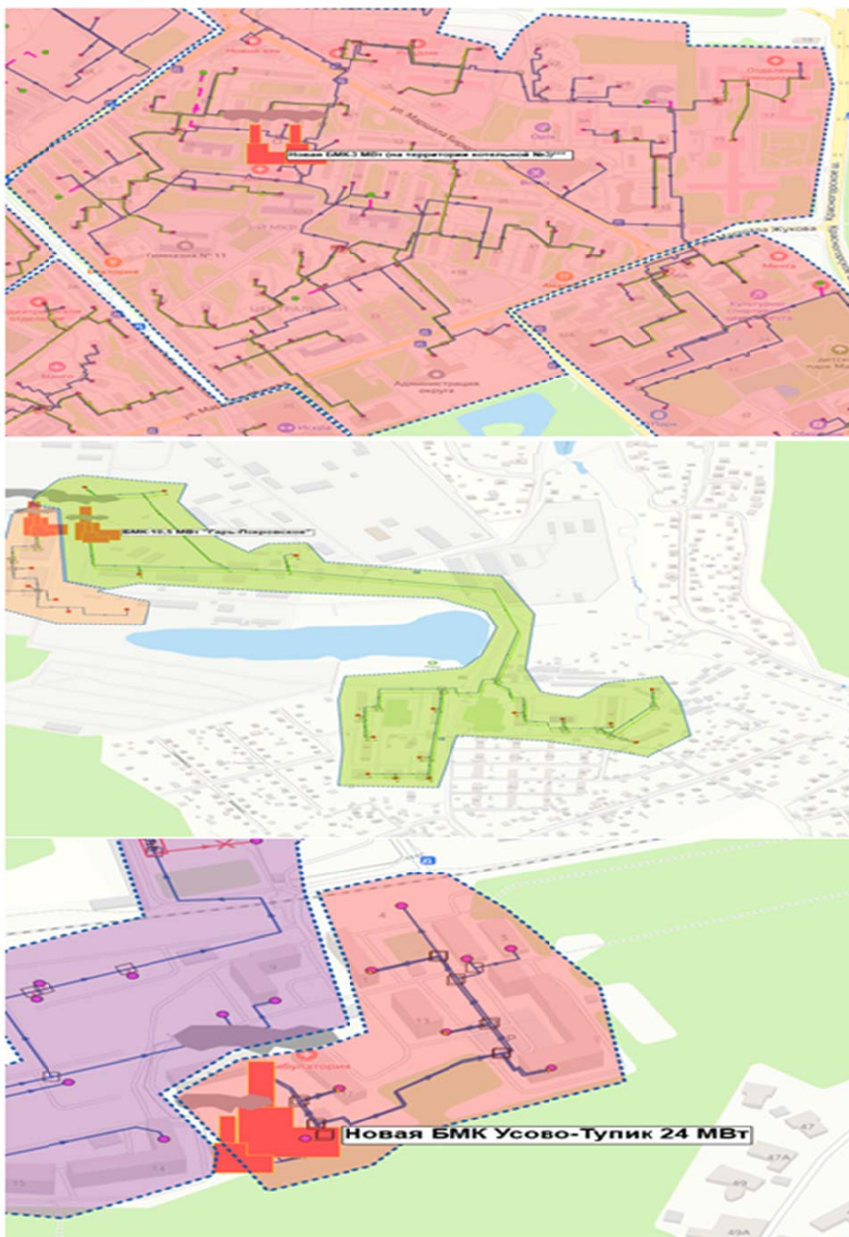
Рисунок 2-8 – Зоны действия перспективных источников централизованного теплоснабжения (продолжение)
