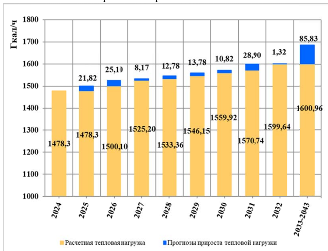
Рисунок 1-2 – Расчетная тепловая нагрузка и прирост тепловой нагрузки на расчетный период
