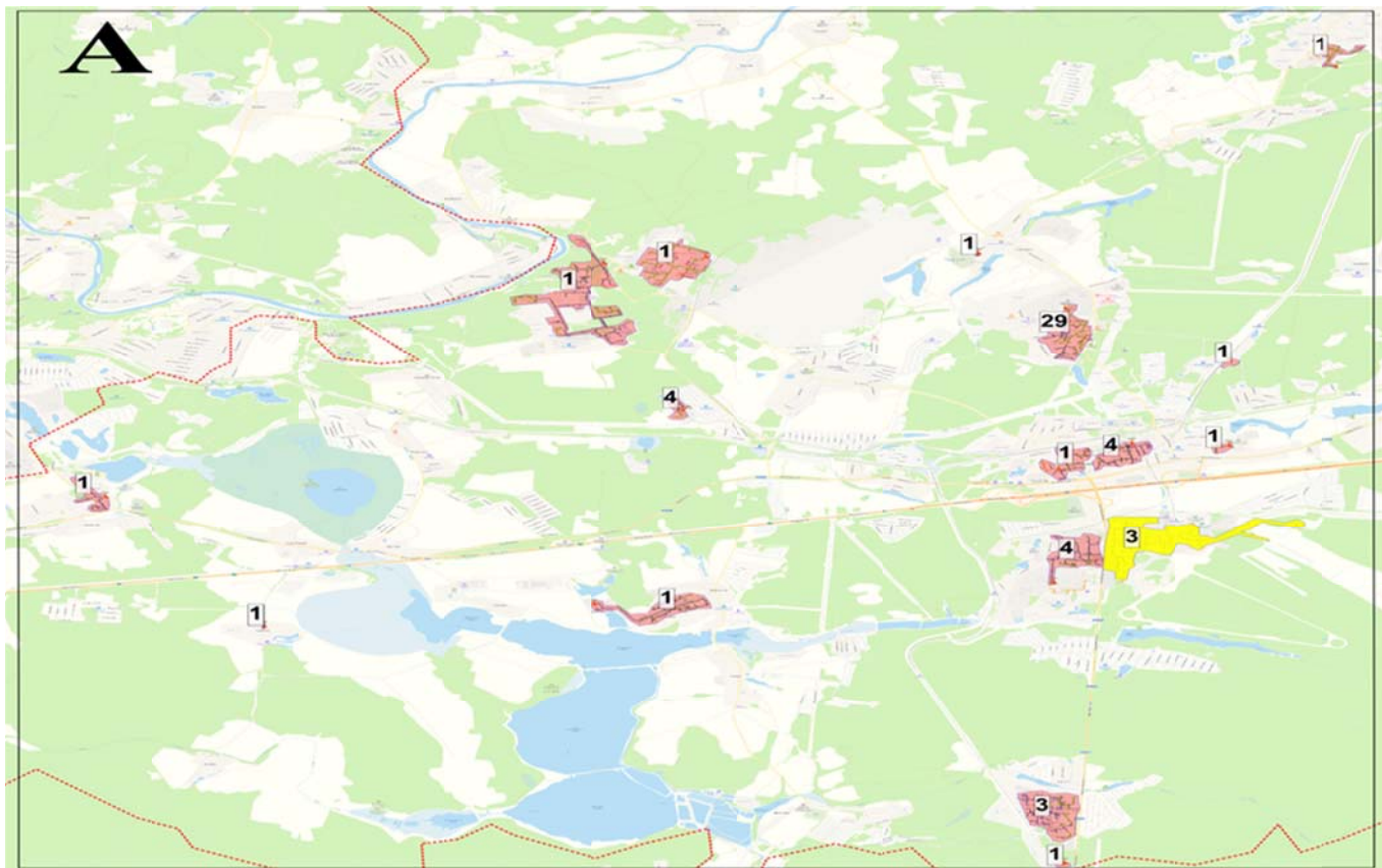
Рисунок 2-2 – Зона А действия источников централизованного теплоснабжения
